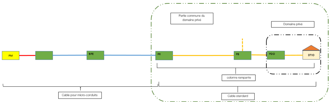
Figure 4 : Schéma de principe PM DTIO zone de logements individuels collectifs (lotissements)
