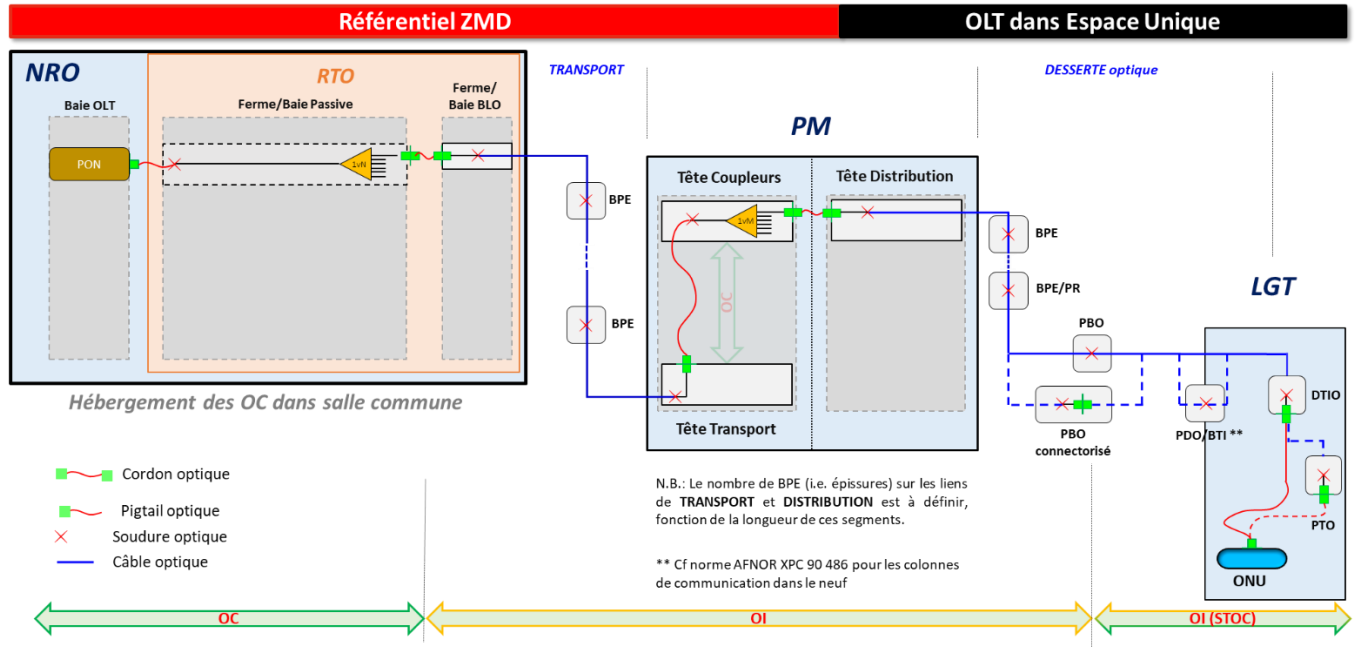
Boucle locale fibre avec l'introduction des nouvelles technologies par ajout d'un élément de coexistence
